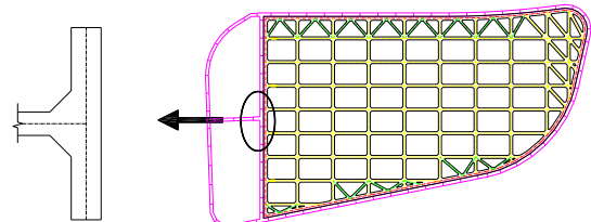
图 3 第一、二道支撑平面布置图 Fig. 3 Plan of the first and second layers of struts
